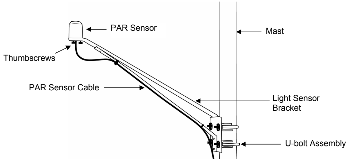
Figure 2: PAR Smart Sensor Bracket Mounting
